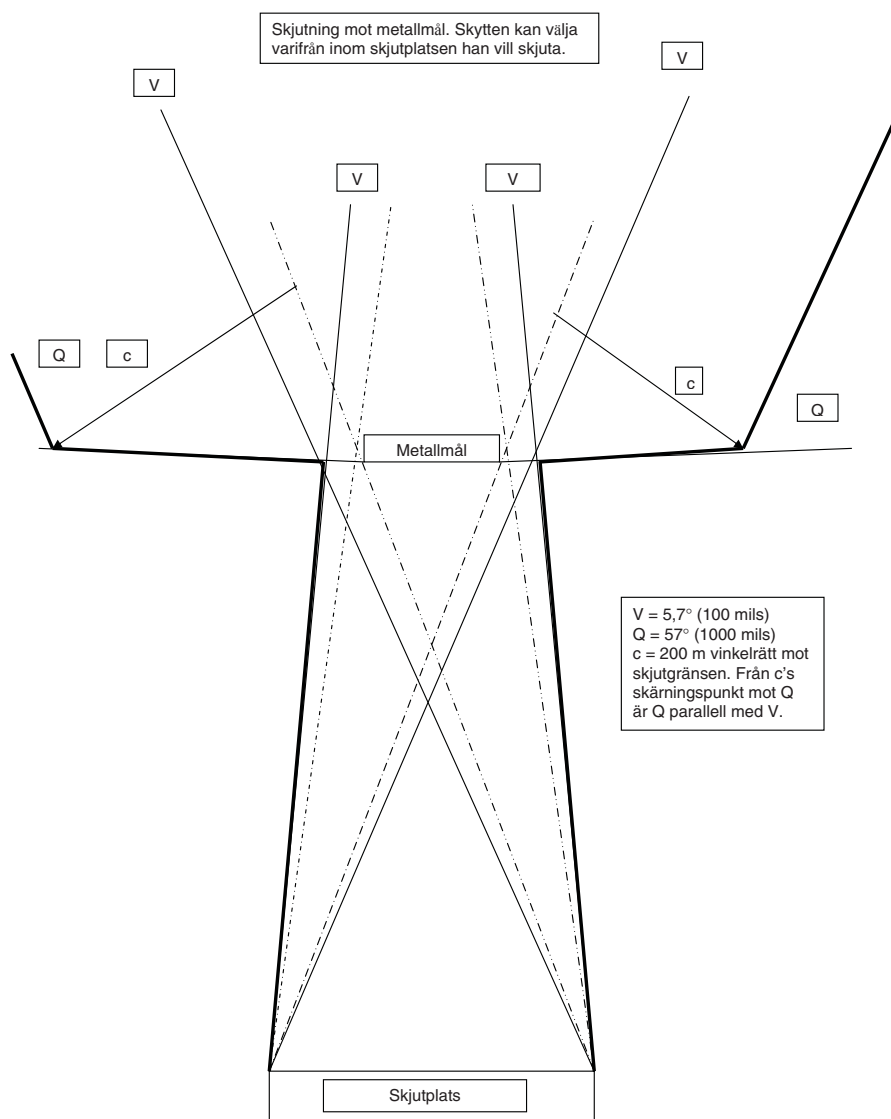
Bild 1: Riskvinklar metallmål
